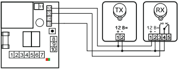
Рис. 6 — Подключение ИК-барьера
