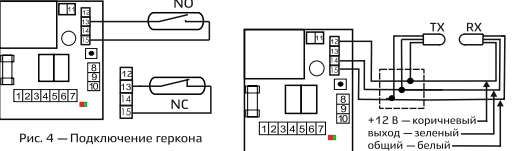
Рис. 4 — Подключение геркона Рис. 5 — Подключение оптосенсора SIGNAL12
