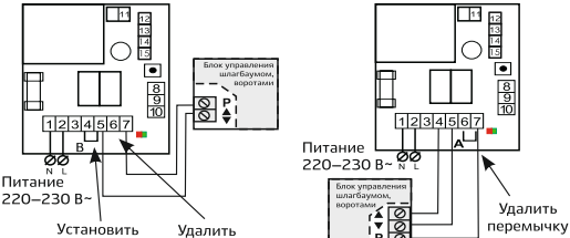
Рис. 2 — Подключение к пошаговому входу Рис. 3 — Подключение к раздельным входам «ОТКРЫТЬ» и «ЗАКРЫТЬ»
