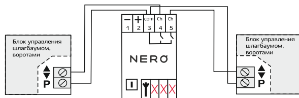
Рис. 3 — Двухканальный режим
