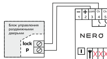
Рис. 4 — Режим непрерывной команды
